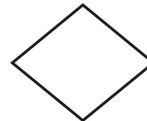
rhombus
